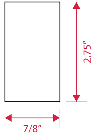
Punchout Dimensions
